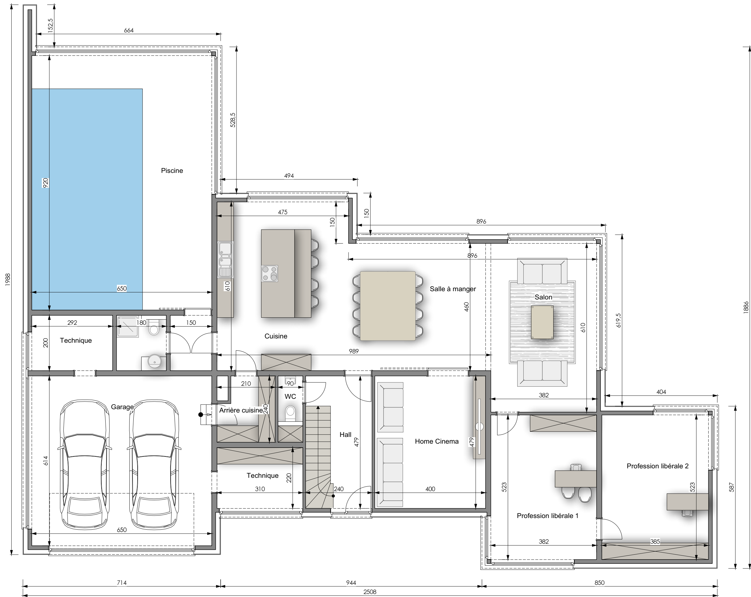
PLAN REZ-DE-CHAUSSEE
