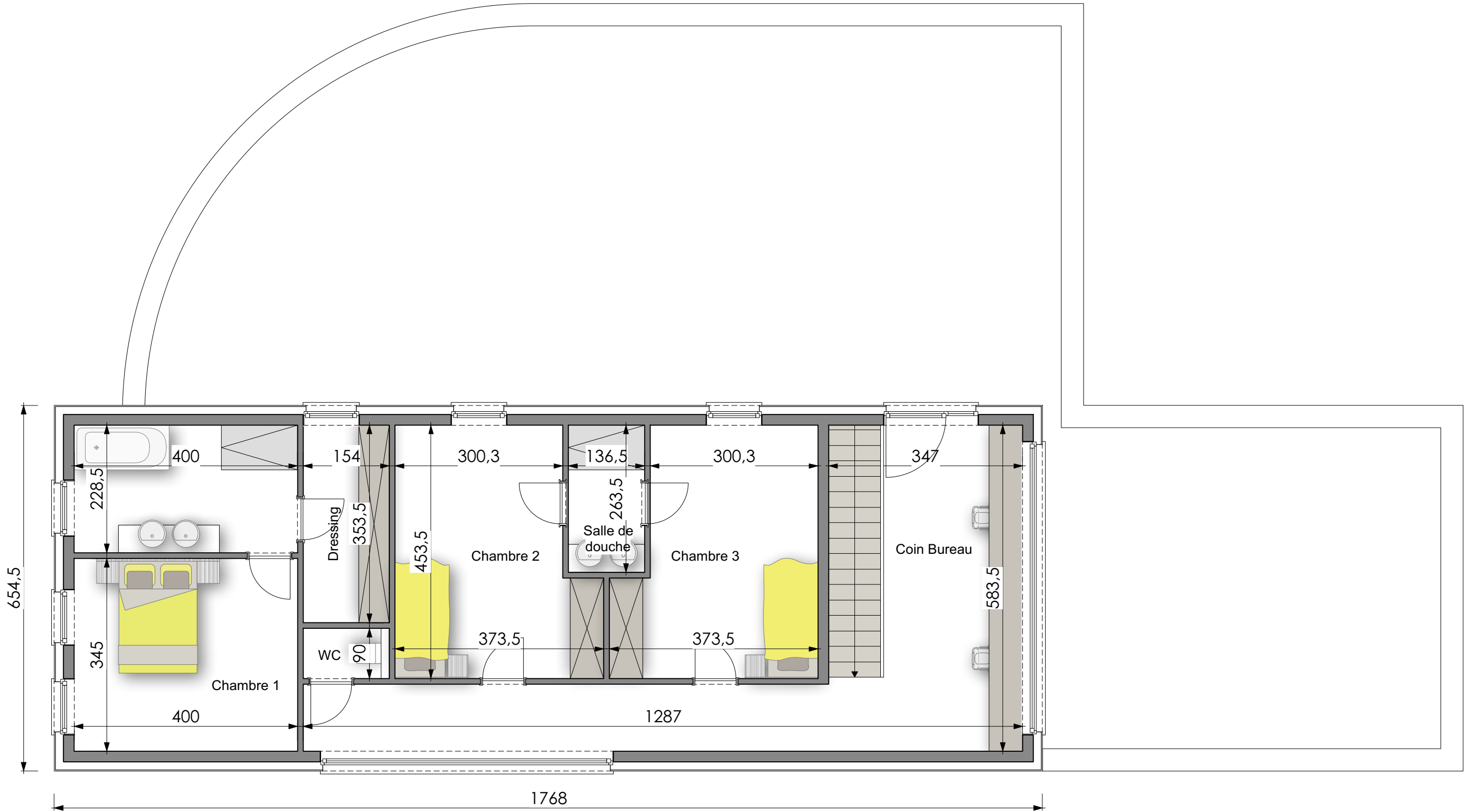
PLAN PREMIER ETAGE
