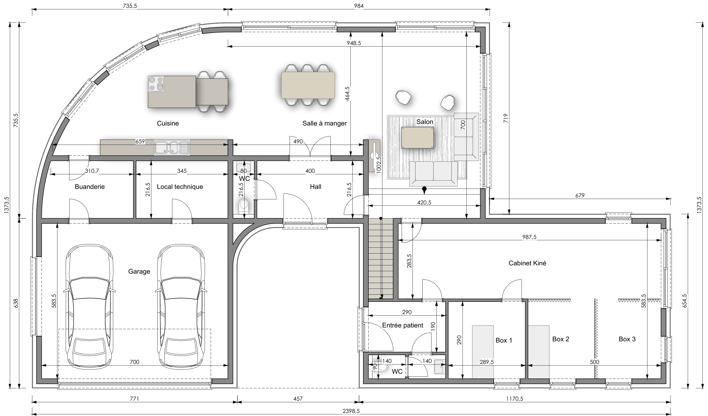
PLAN REZ-DE-CHAUSSEE
