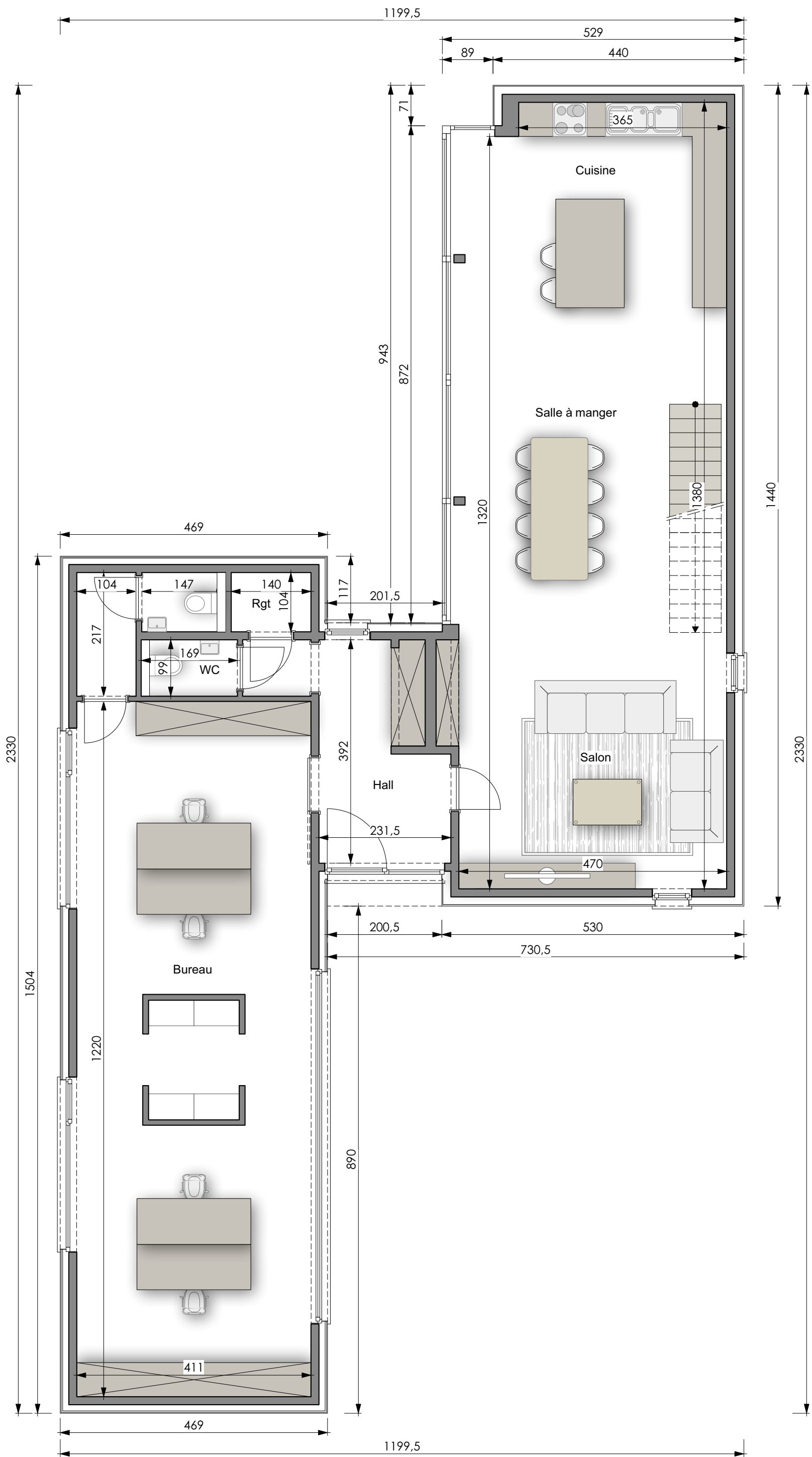
PLAN REZ-DE-CHAUSSEE
