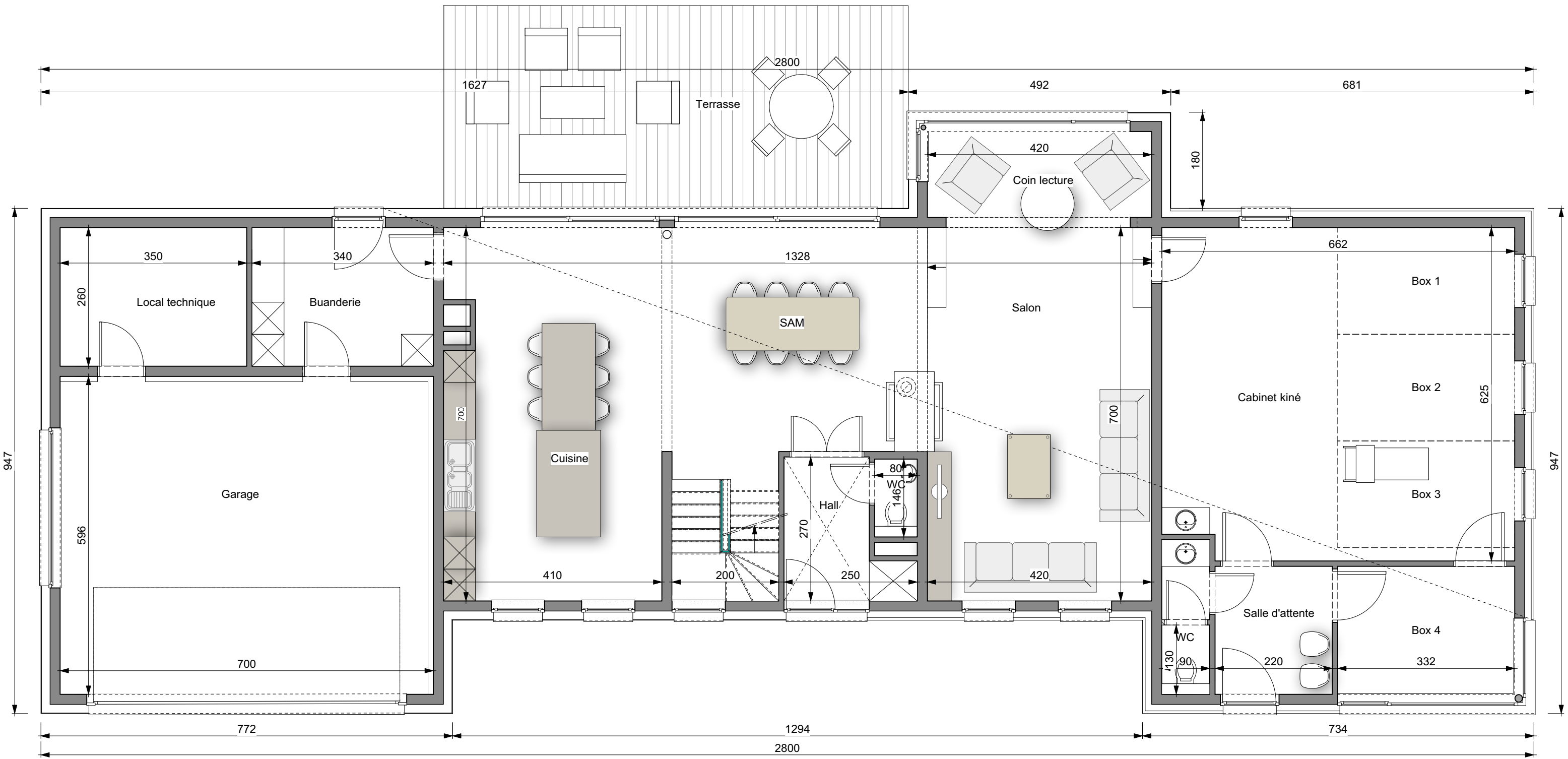
PLAN REZ-DE-CHAUSSEE
