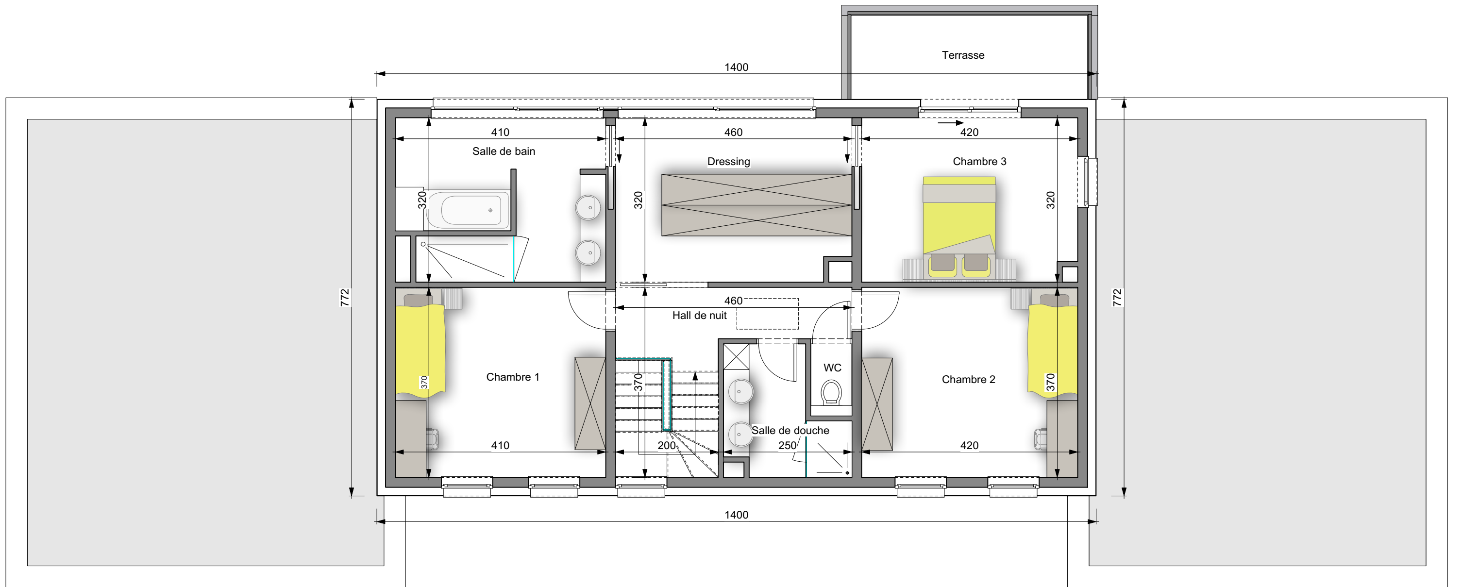
PLAN PREMIER ETAGE
