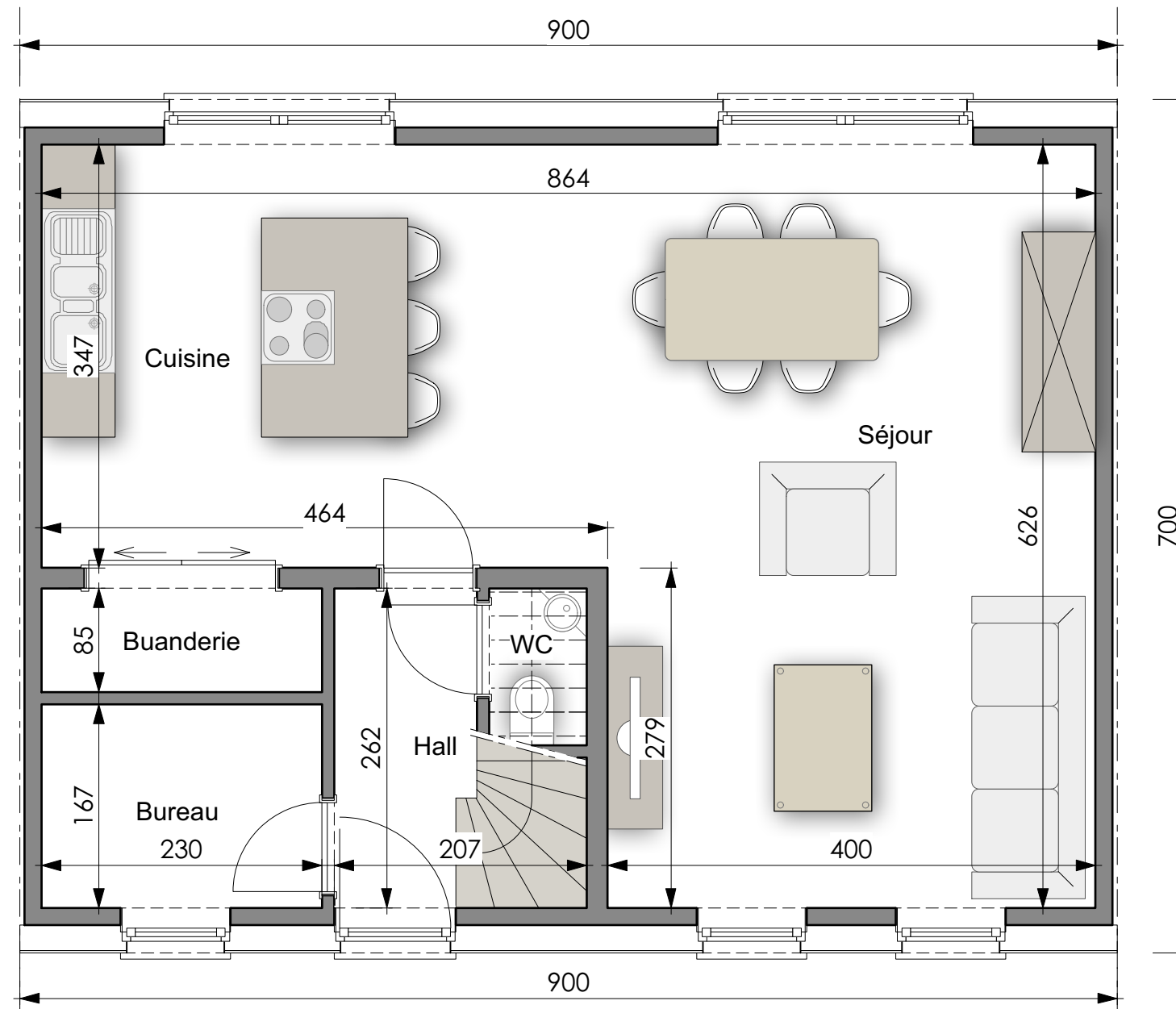
PLAN REZ-DE-CHAUSSEE
