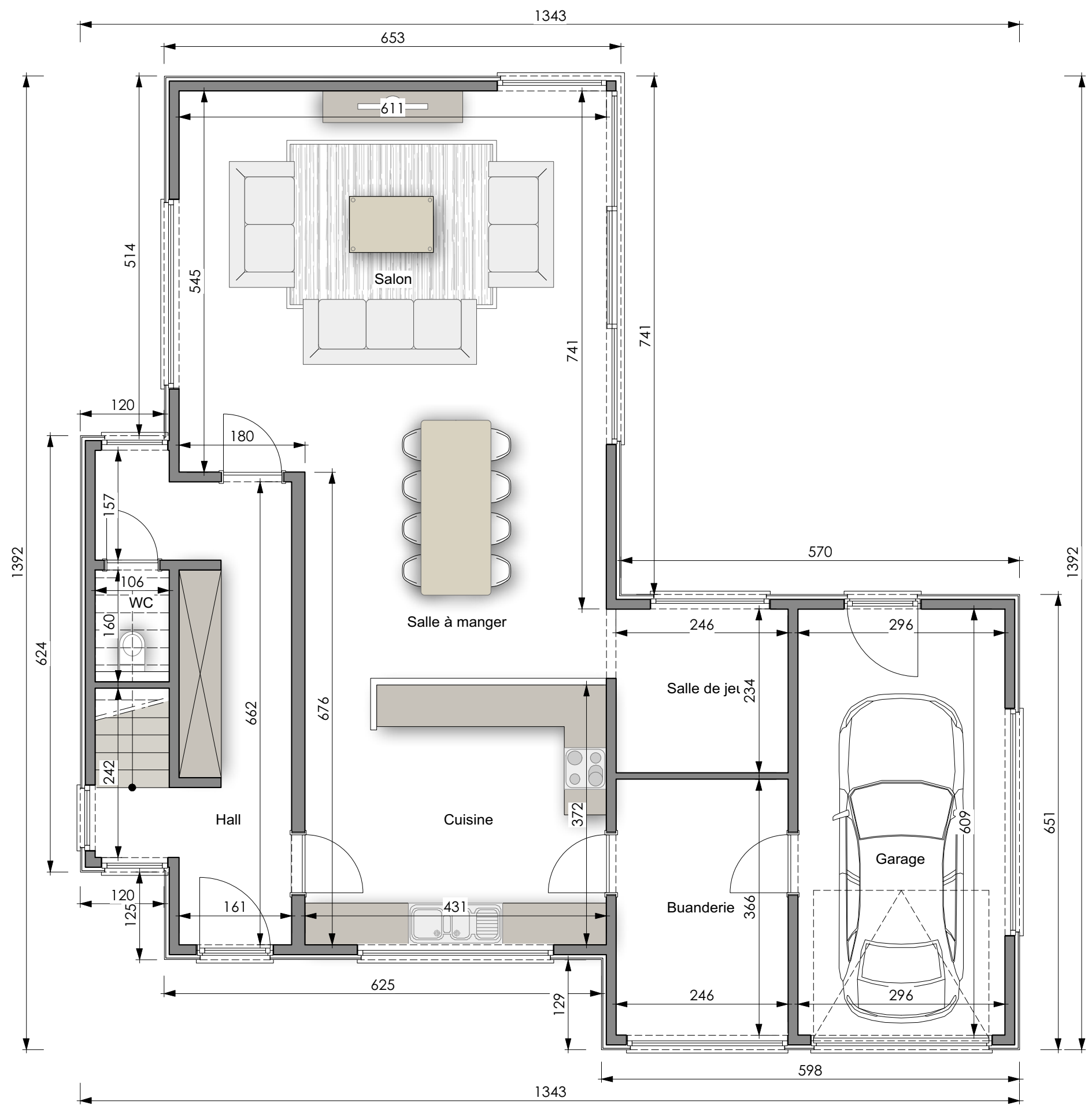
PLAN REZ-DE-CHAUSSEE
