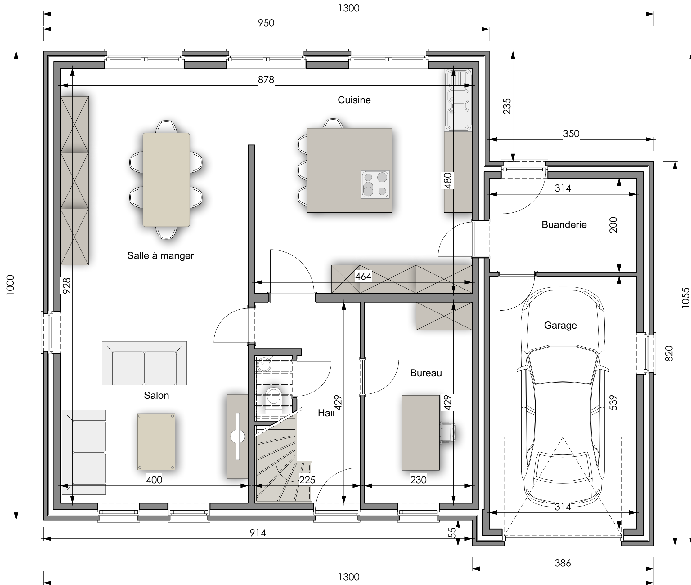
PLAN REZ-DE-CHAUSSEE
