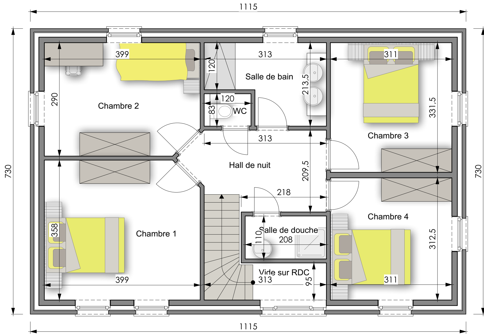
PLAN PREMIER ETAGE
