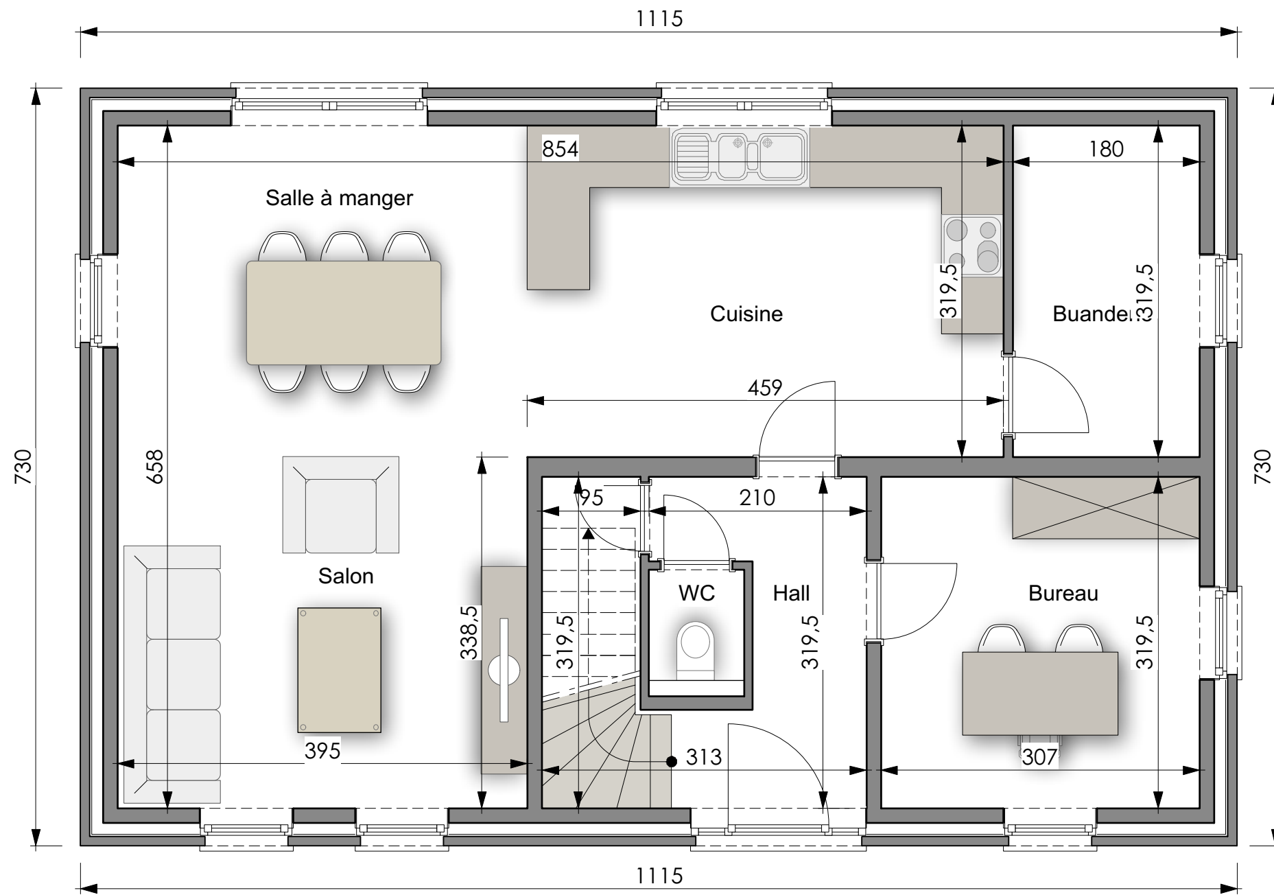
PLAN REZ-DE-CHAUSSEE
