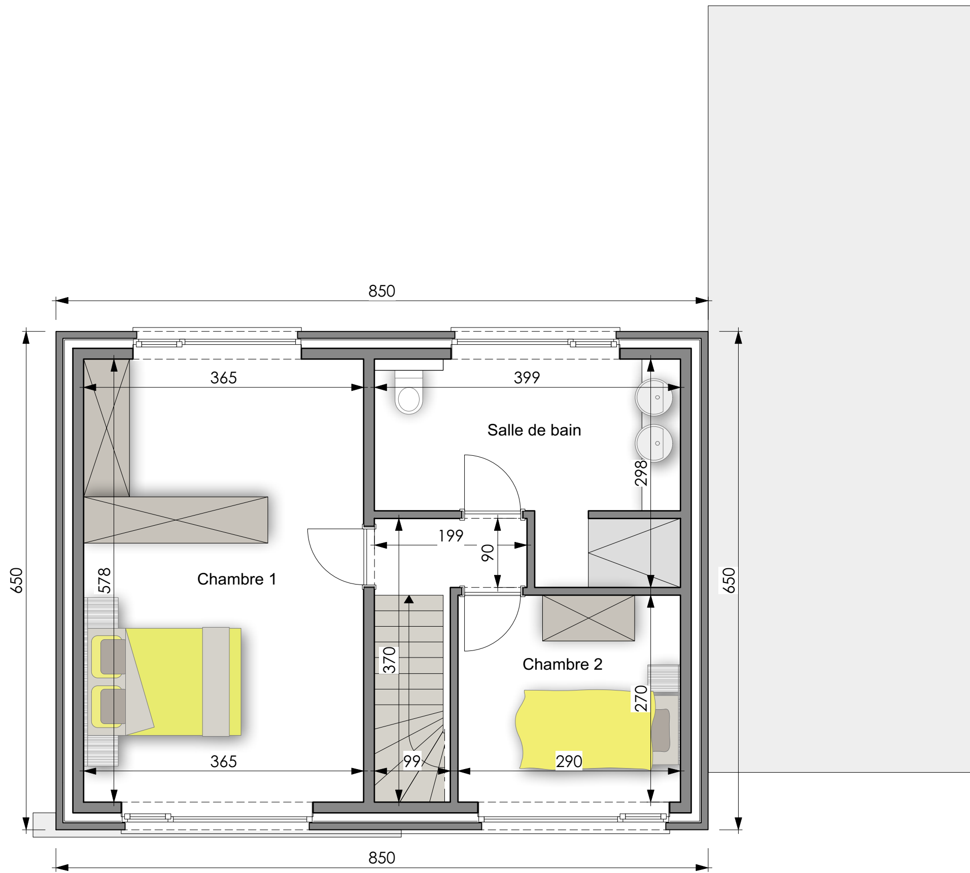
PLAN PREMIER ETAGE
