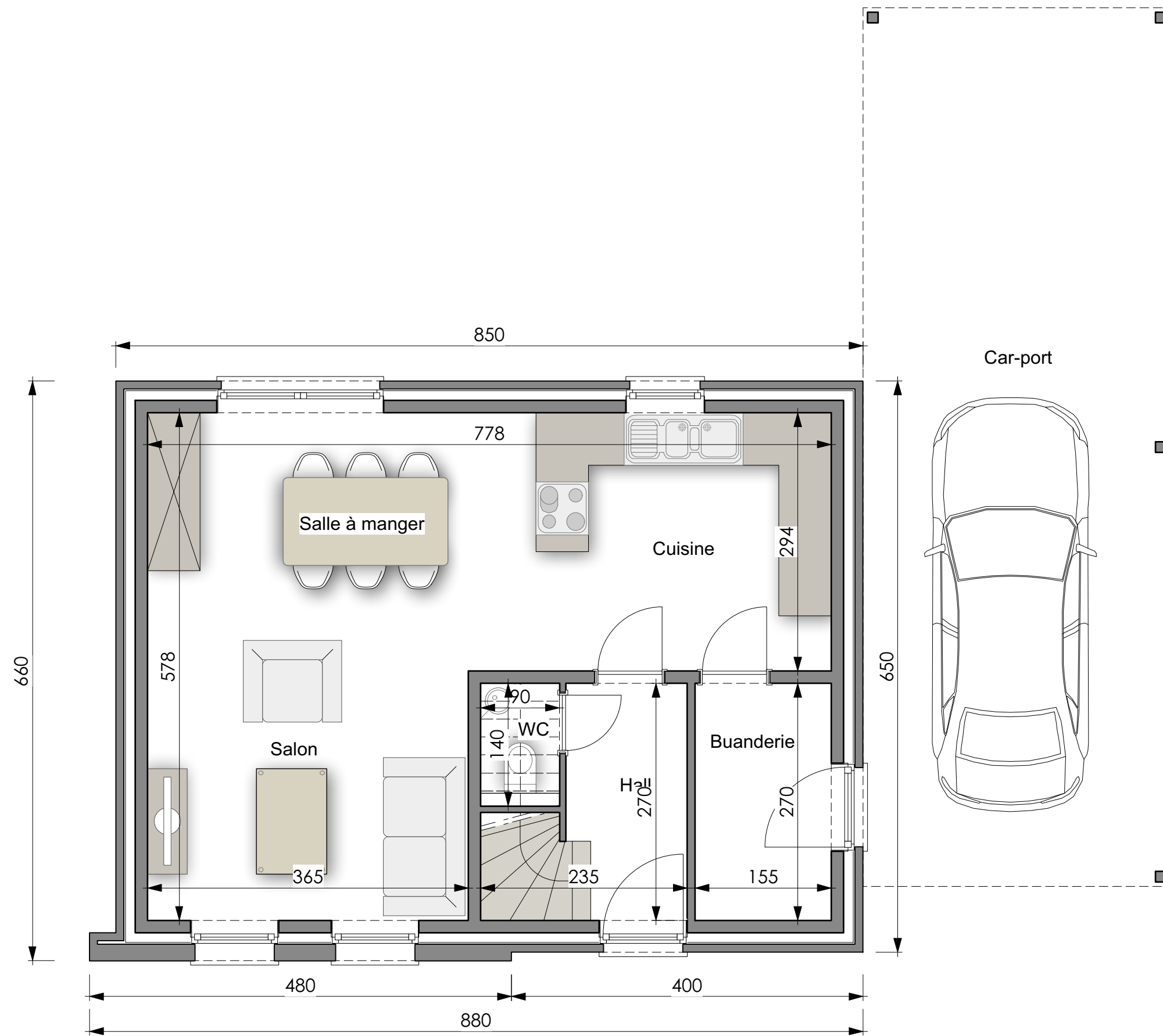
PLAN REZ-DE-CHAUSSEE
