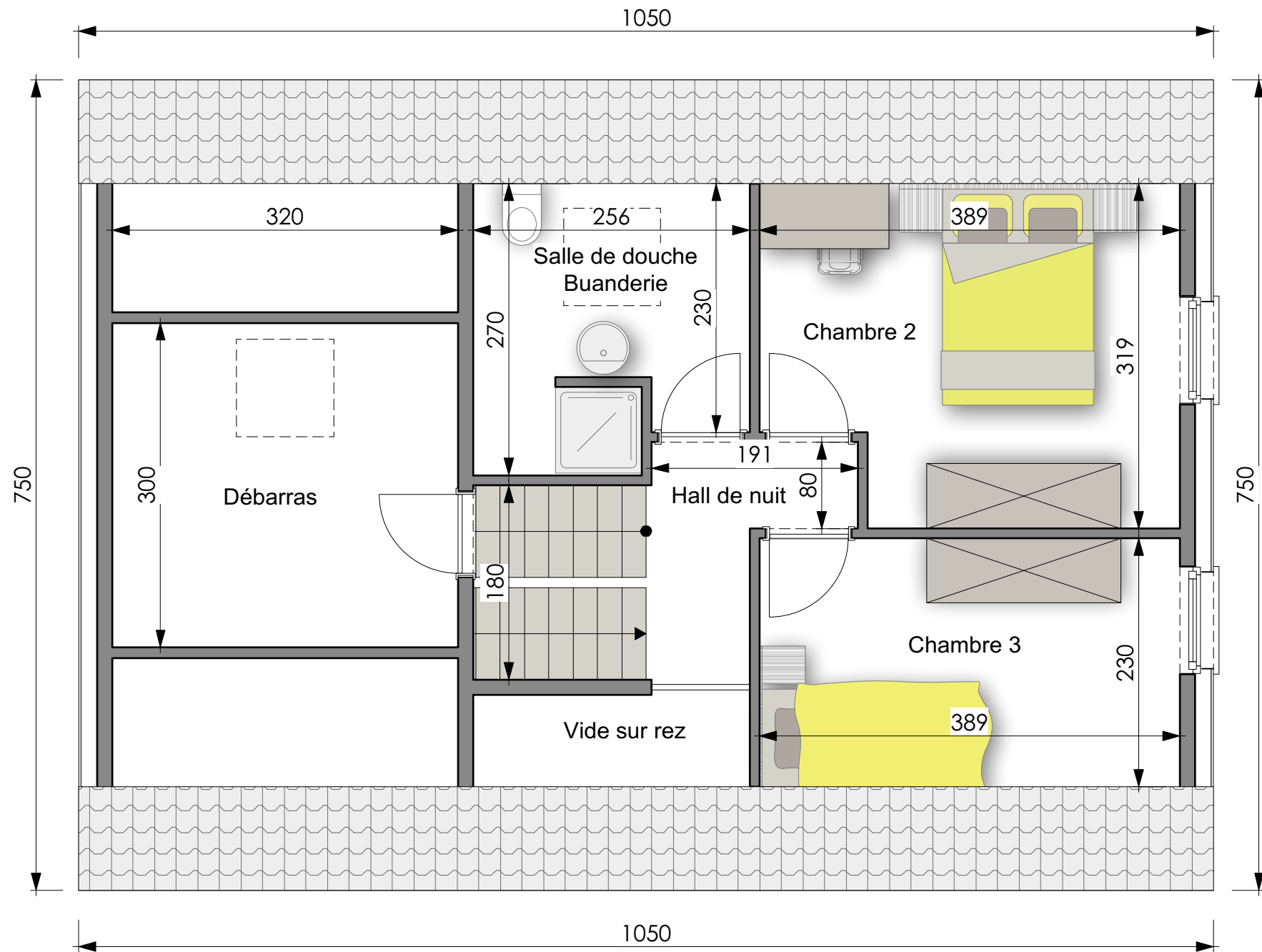
PLAN PREMIER ETAGE
