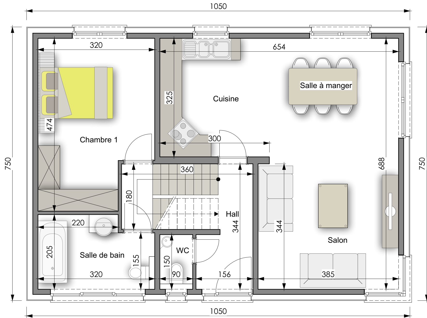
PLAN REZ-DE-CHAUSSEE
