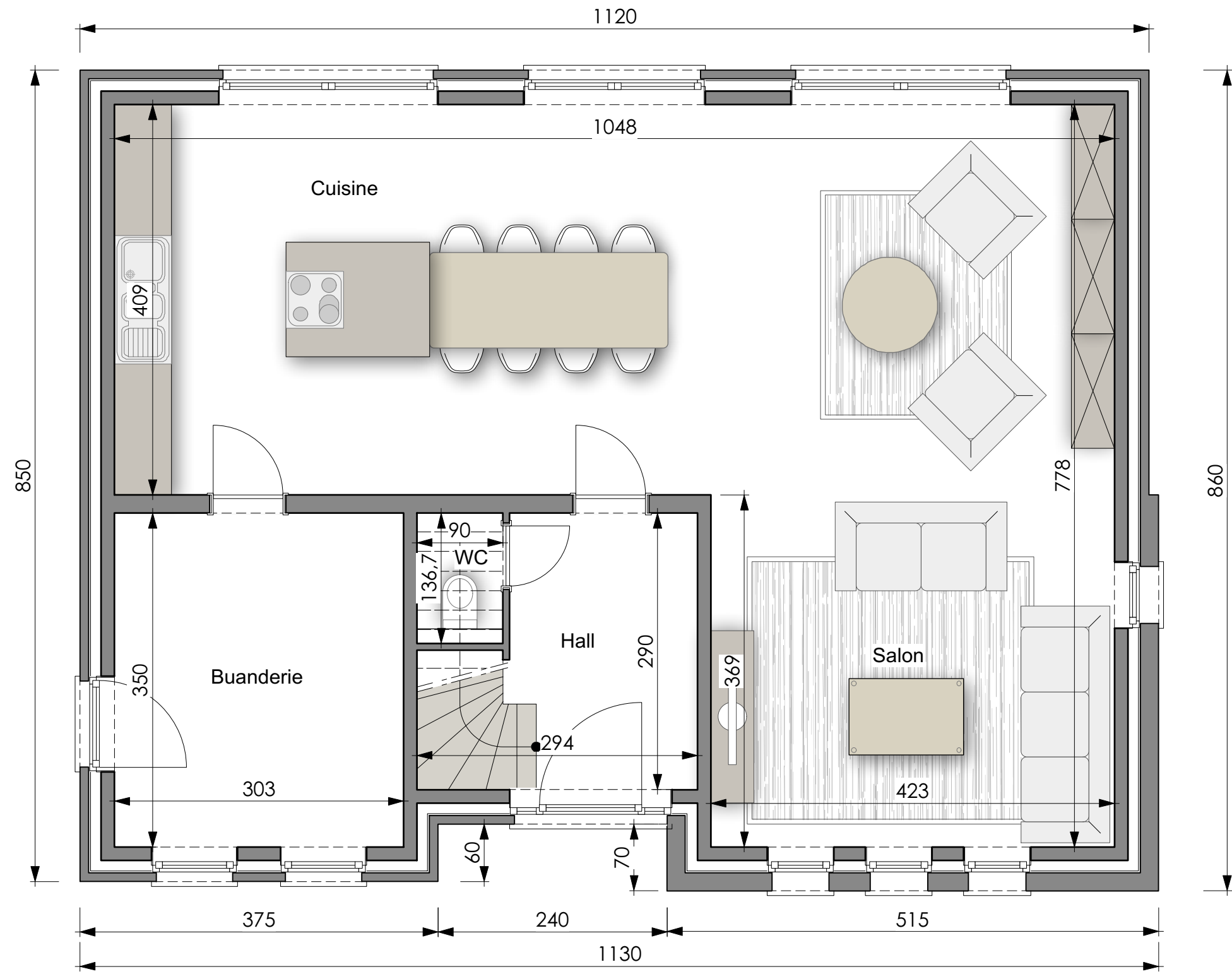
PLAN REZ-DE-CHAUSSEE
