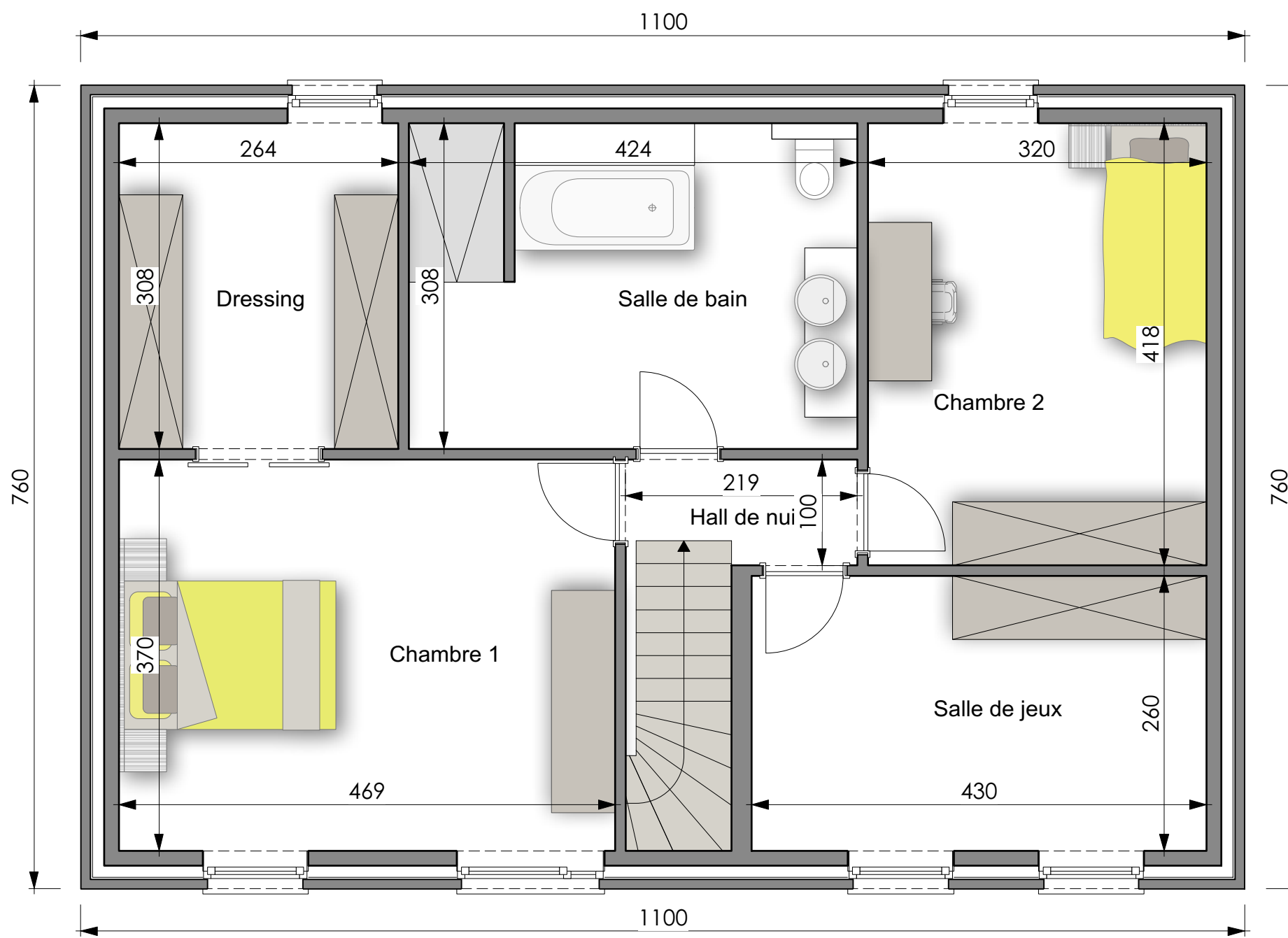
PLAN PREMIER ETAGE
