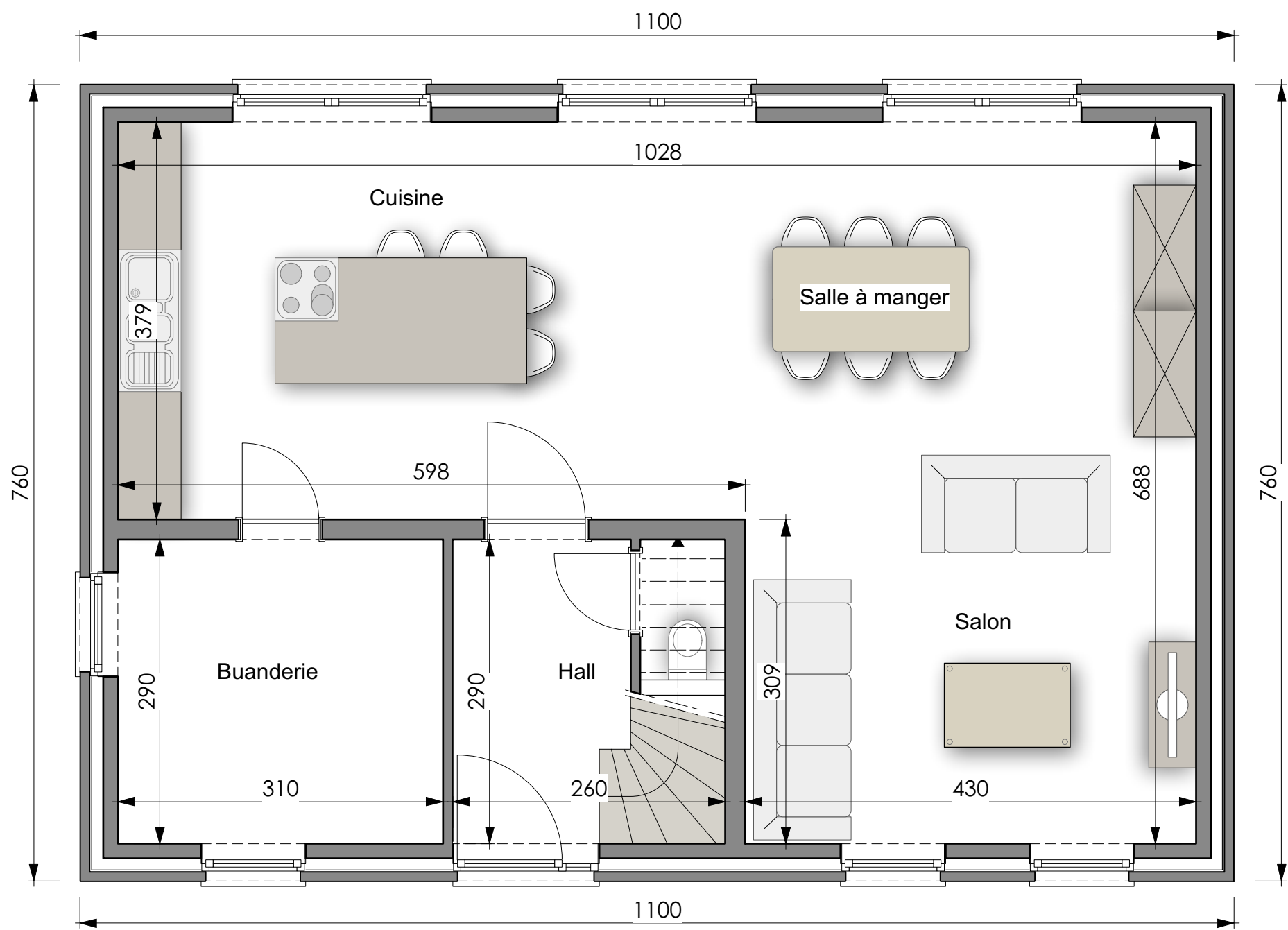
PLAN REZ-DE-CHAUSSEE
