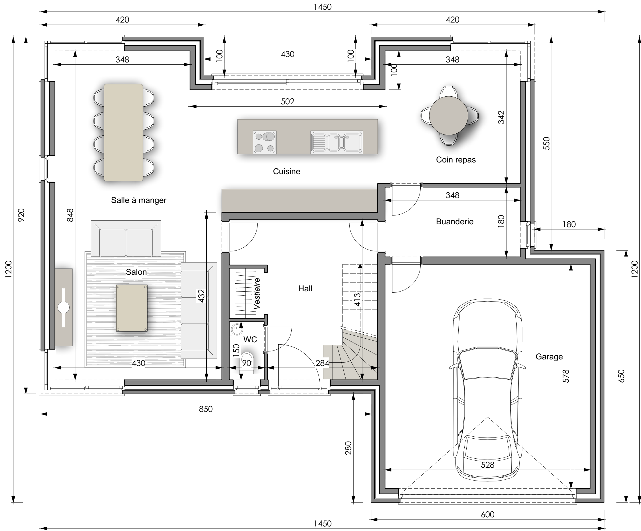
PLAN REZ-DE-CHAUSSEE
