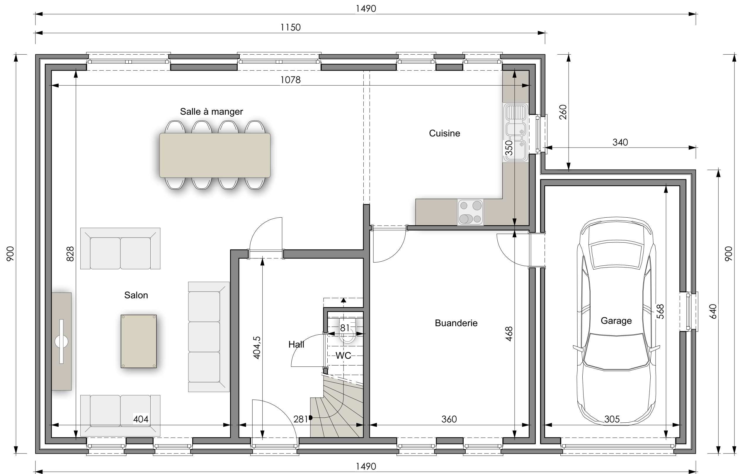
PLAN REZ-DE-CHAUSSEE
