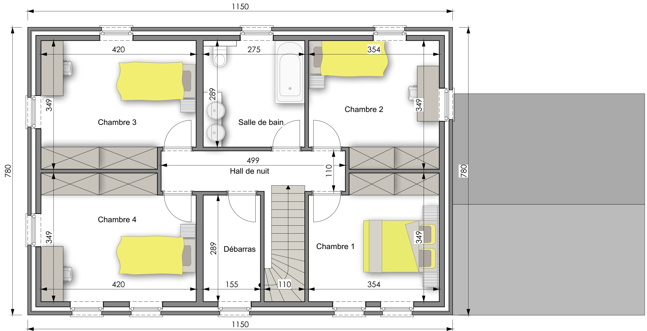
PLAN PREMIER ETAGE
