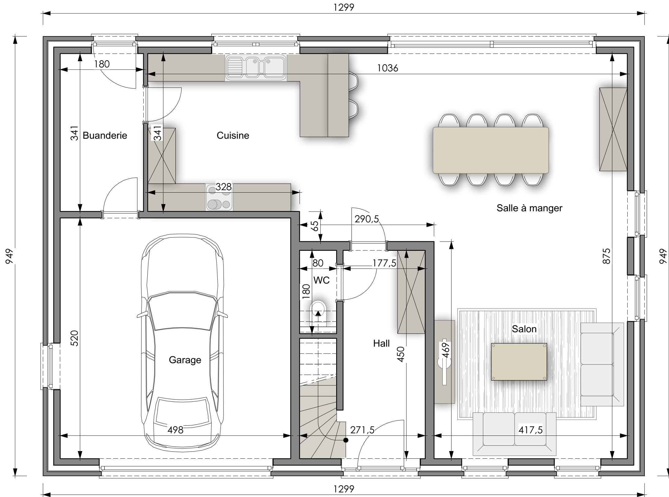
PLAN REZ-DE-CHAUSSEE
