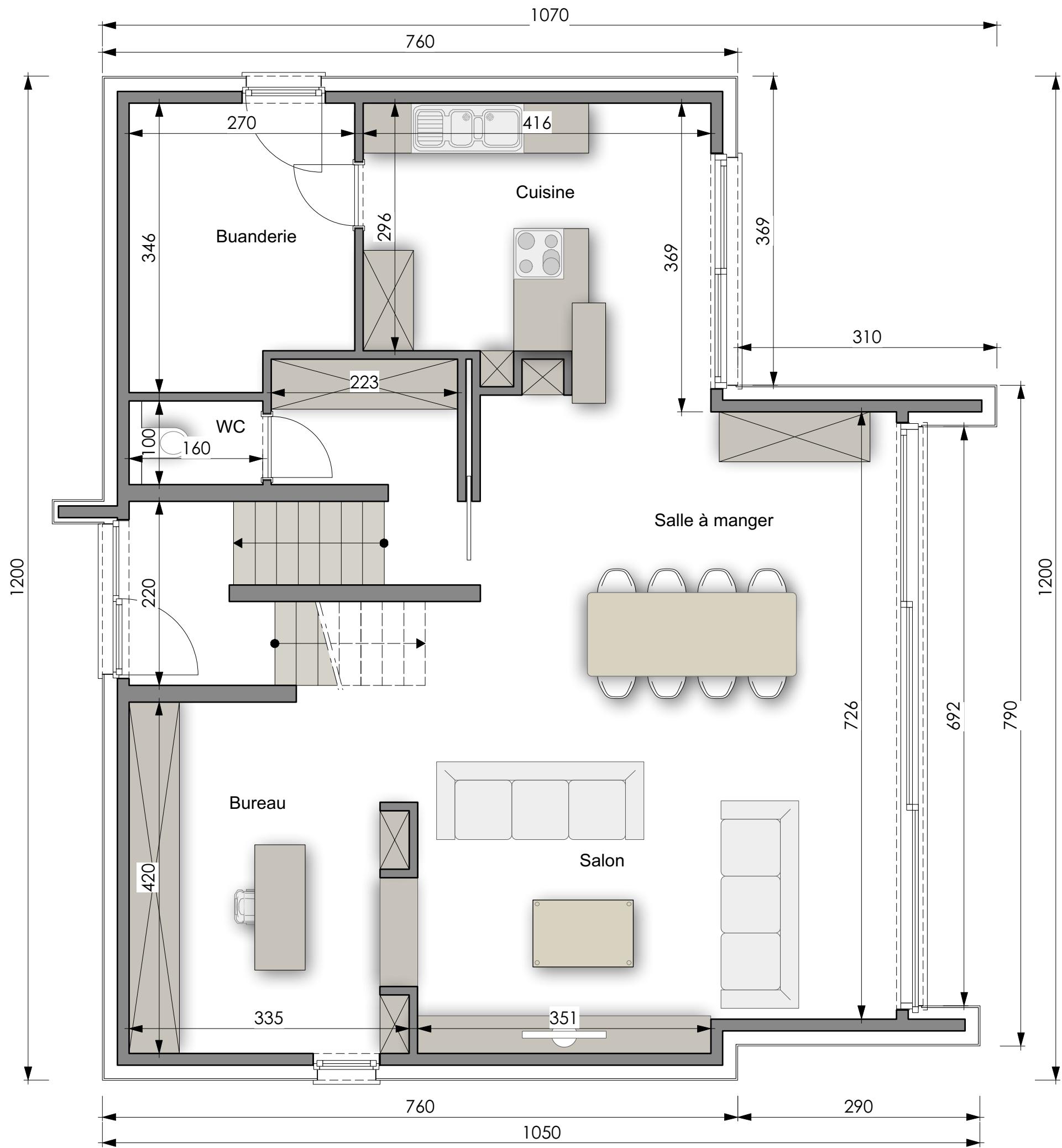
PLAN REZ-DE-CHAUSSEE
