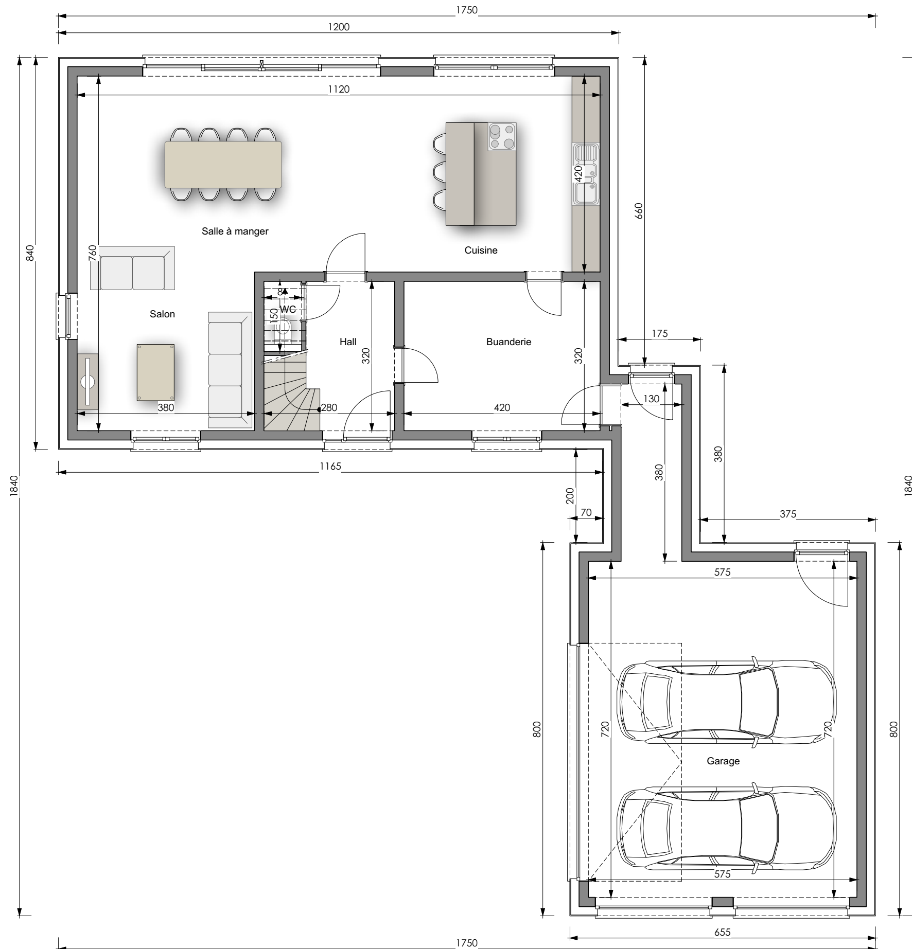
PLAN REZ-DE-CHAUSSEE
