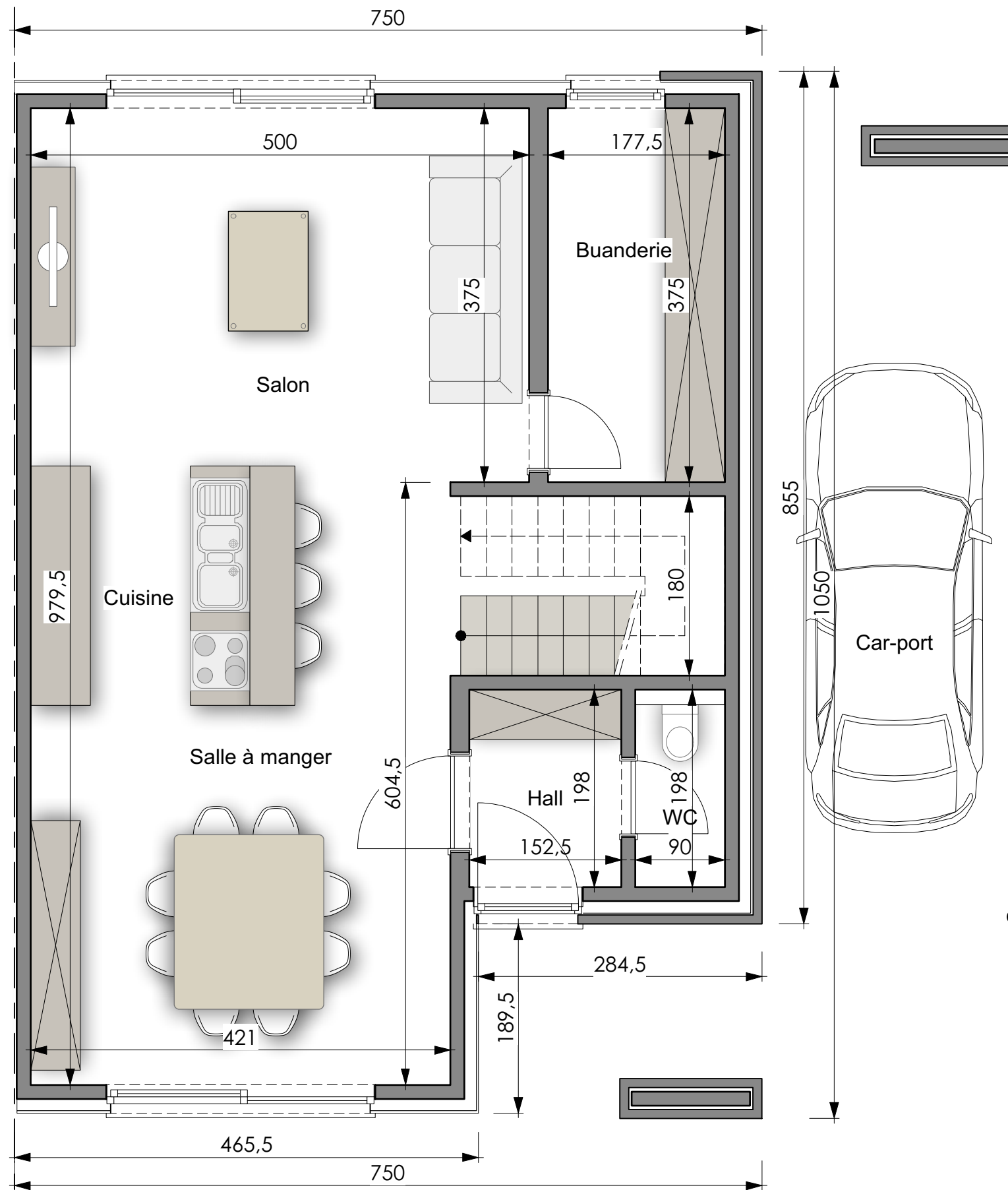
PLAN REZ-DE-CHAUSSEE
