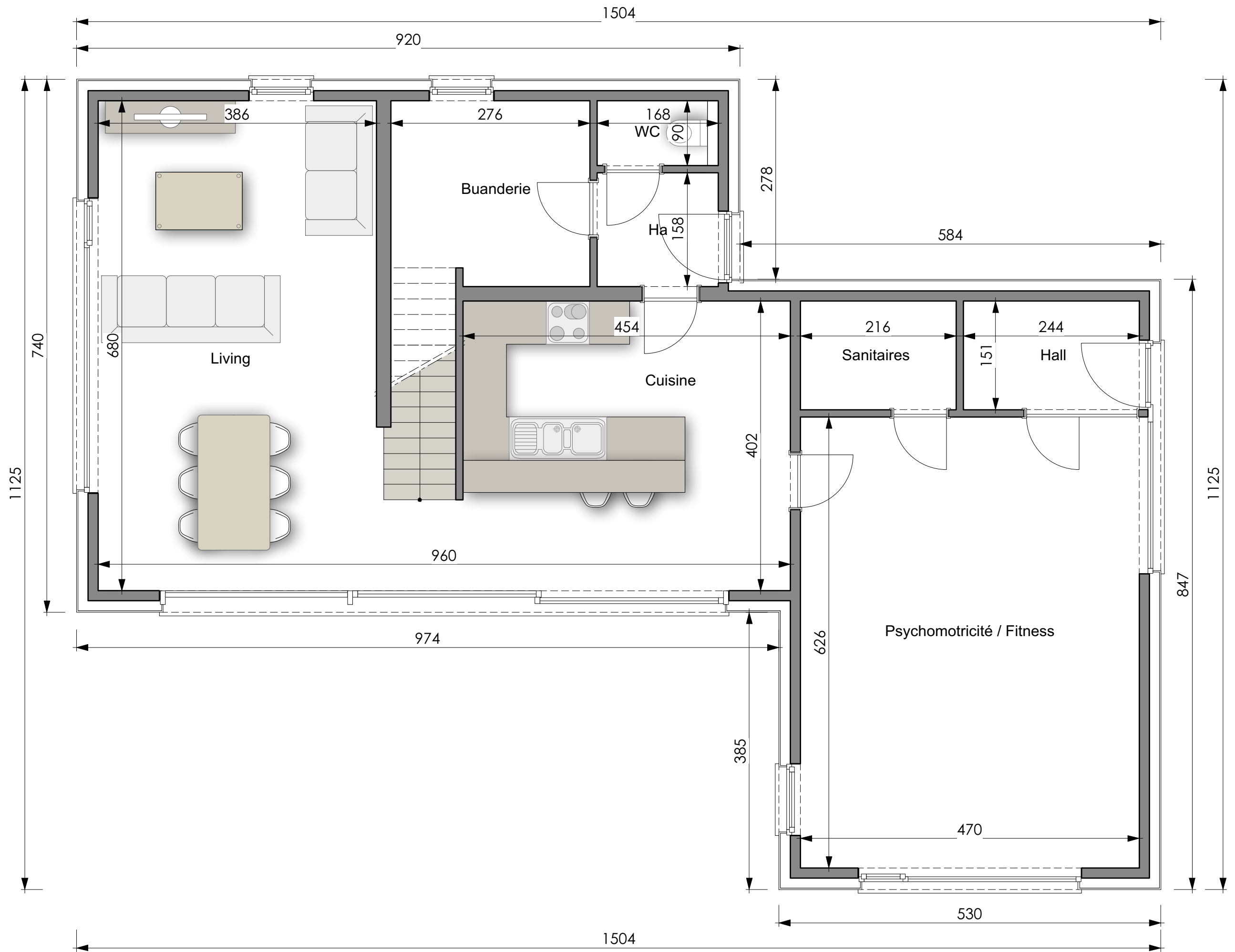
PLAN REZ-DE-CHAUSSEE
