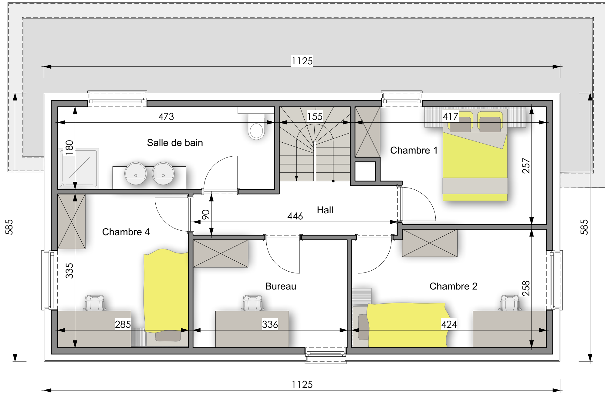
PLAN PREMIER ETAGE
