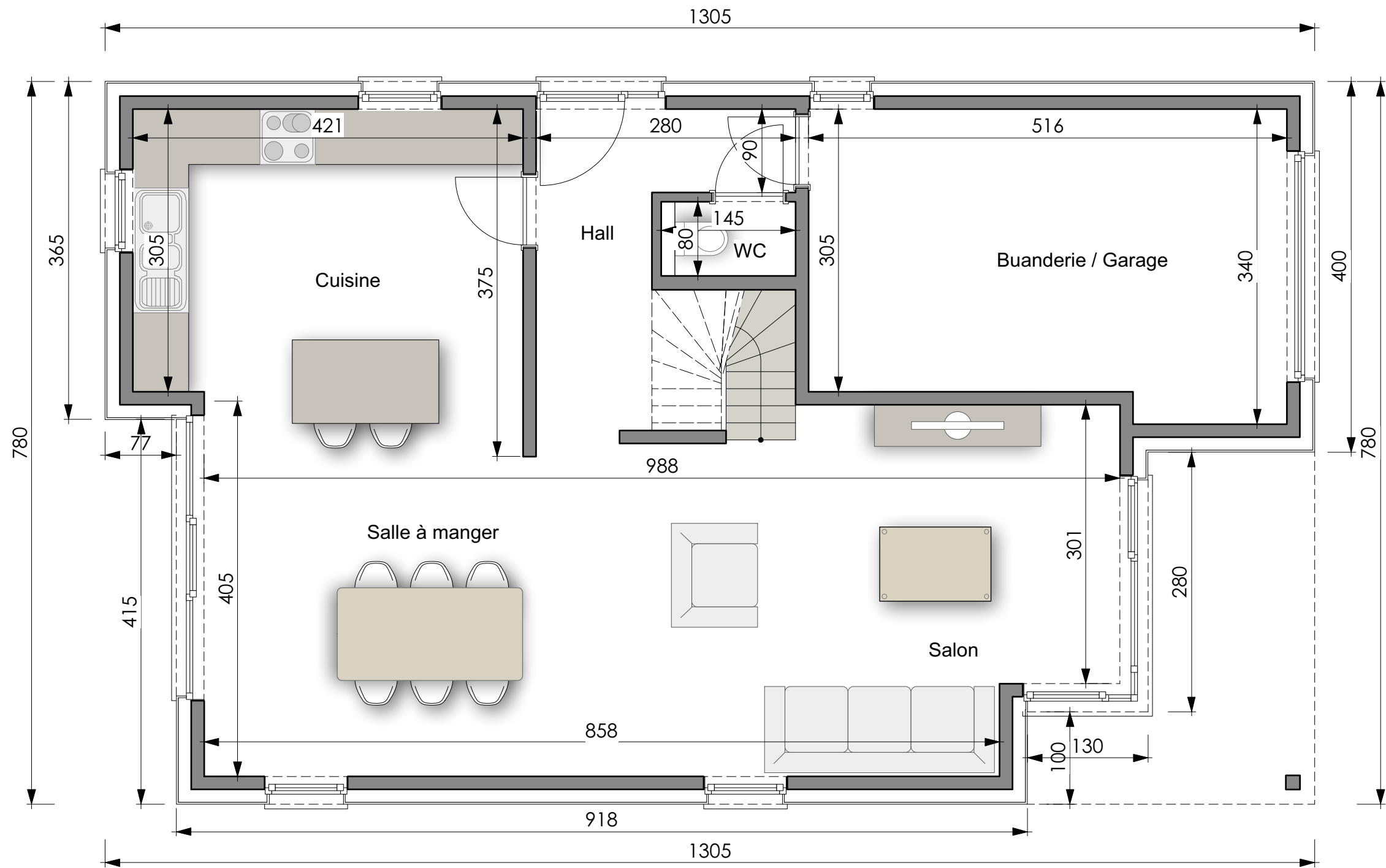
PLAN REZ-DE-CHAUSSEE
