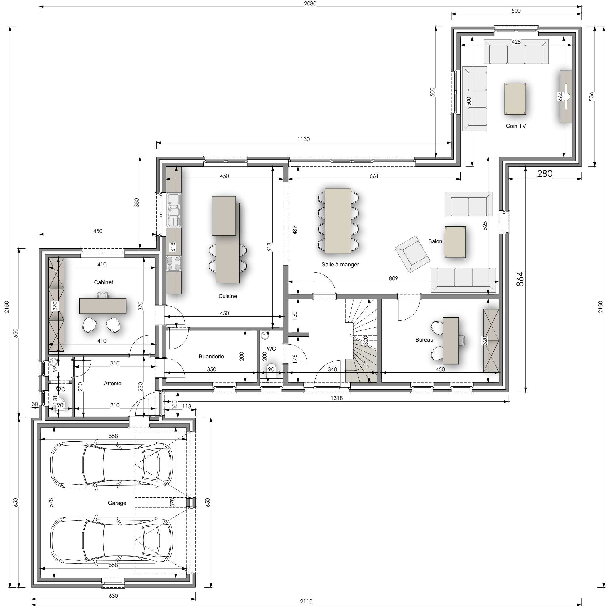
PLAN REZ-DE-CHAUSSEE
