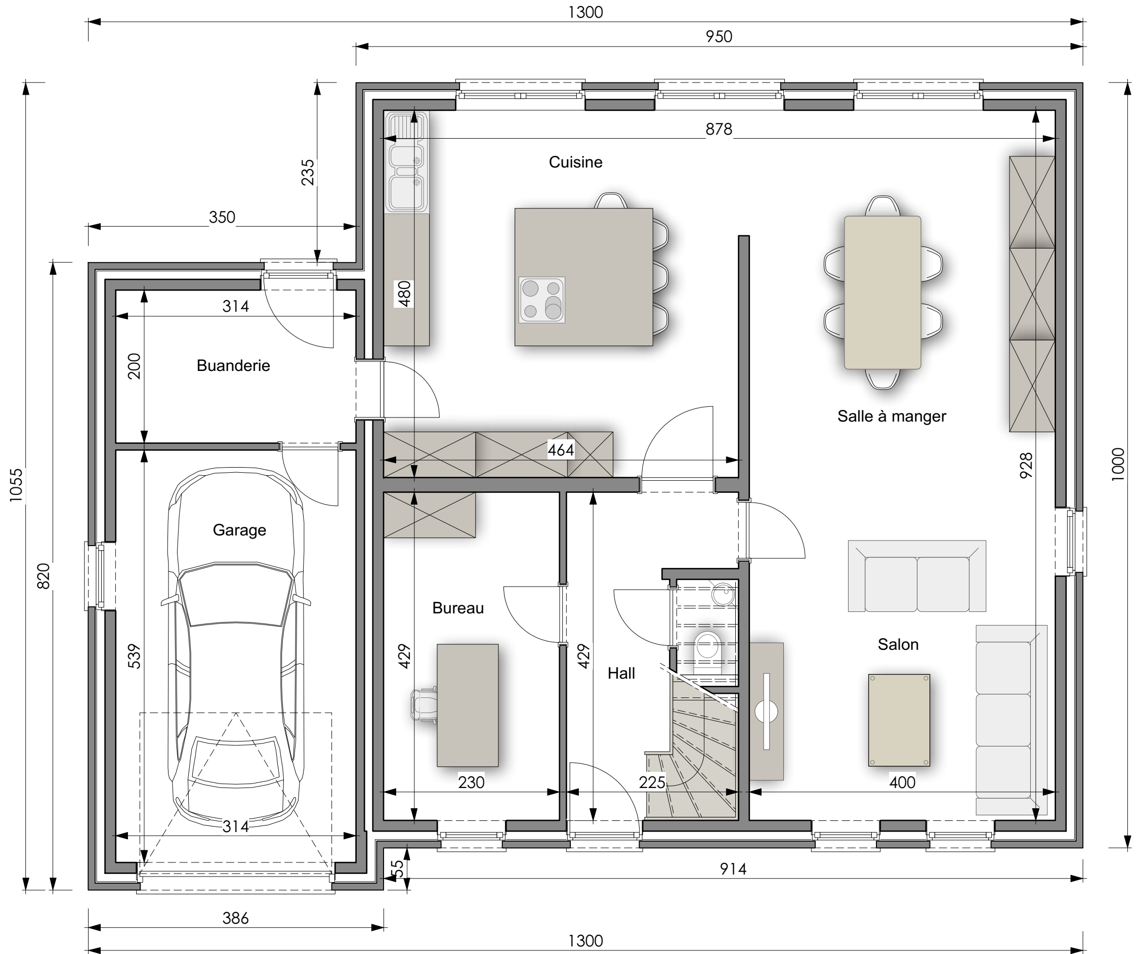
PLAN REZ-DE-CHAUSSEE
