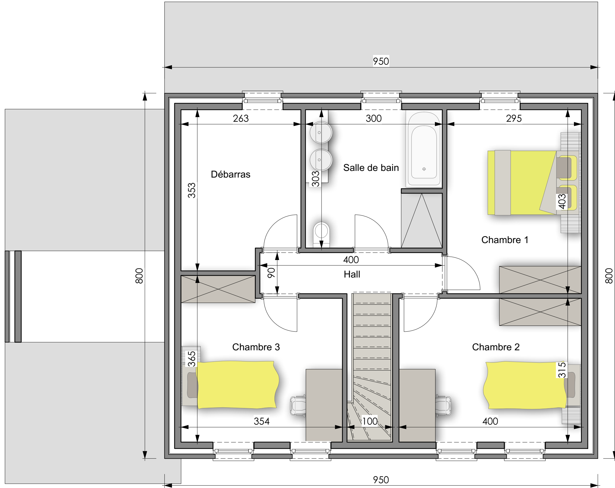
PLAN PREMIER ETAGE
