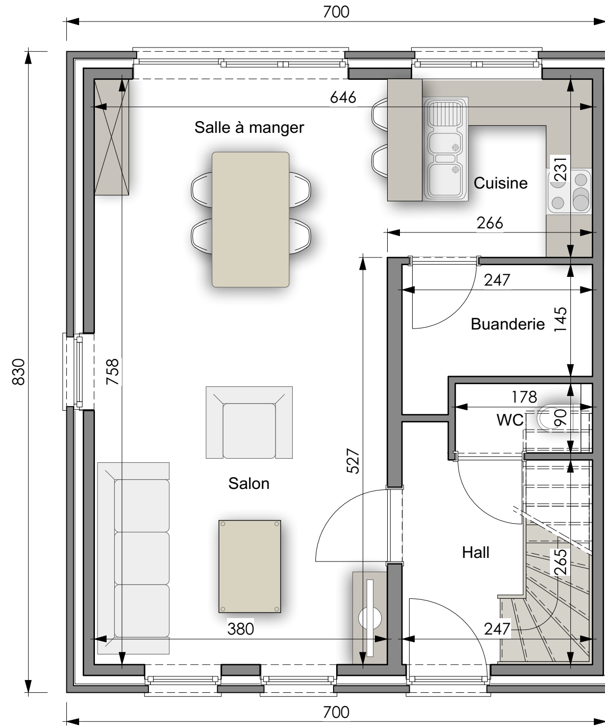
PLAN REZ-DE-CHAUSSEE
