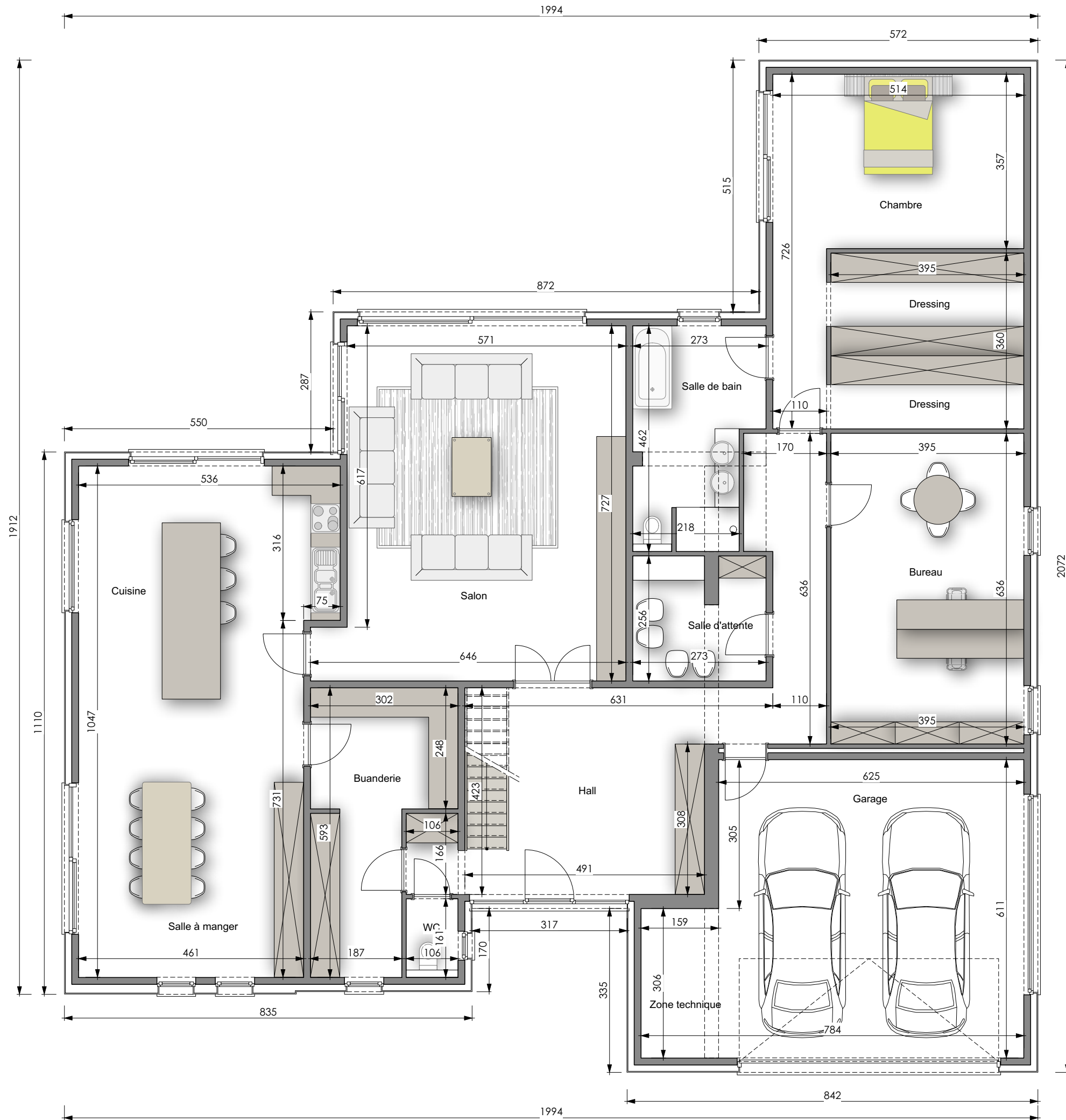
PLAN REZ-DE-CHAUSSEE
