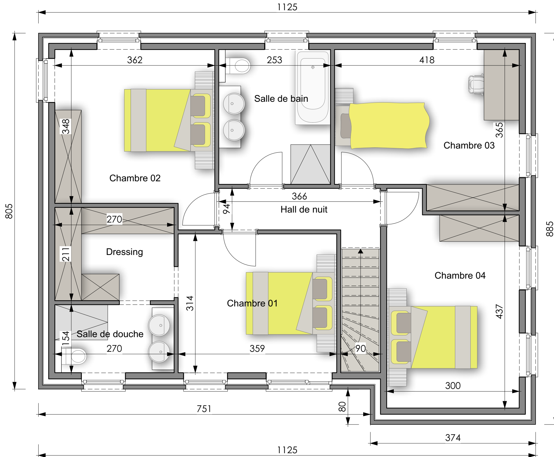
PLAN PREMIER ETAGE
