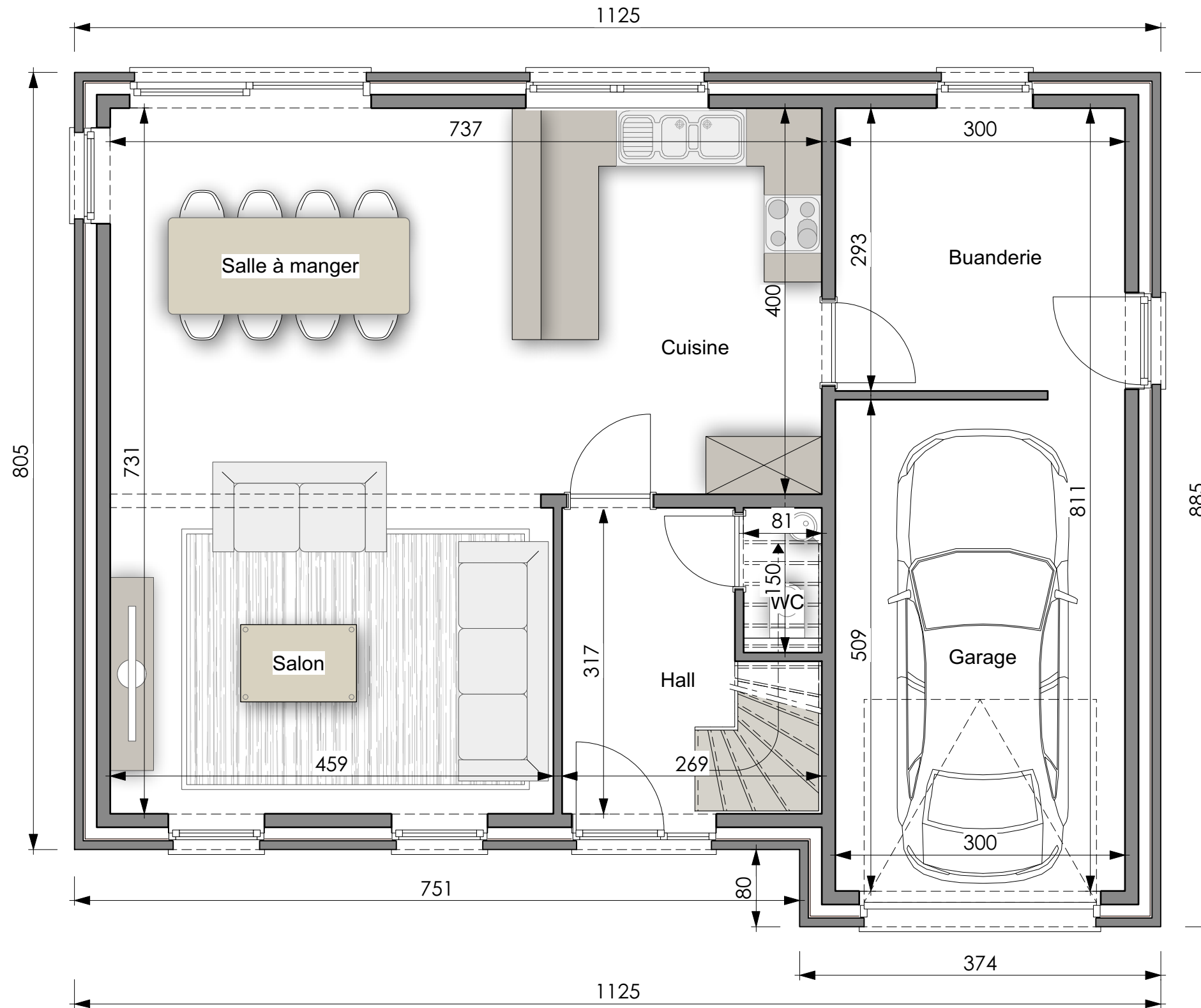
PLAN REZ-DE-CHAUSSEE
