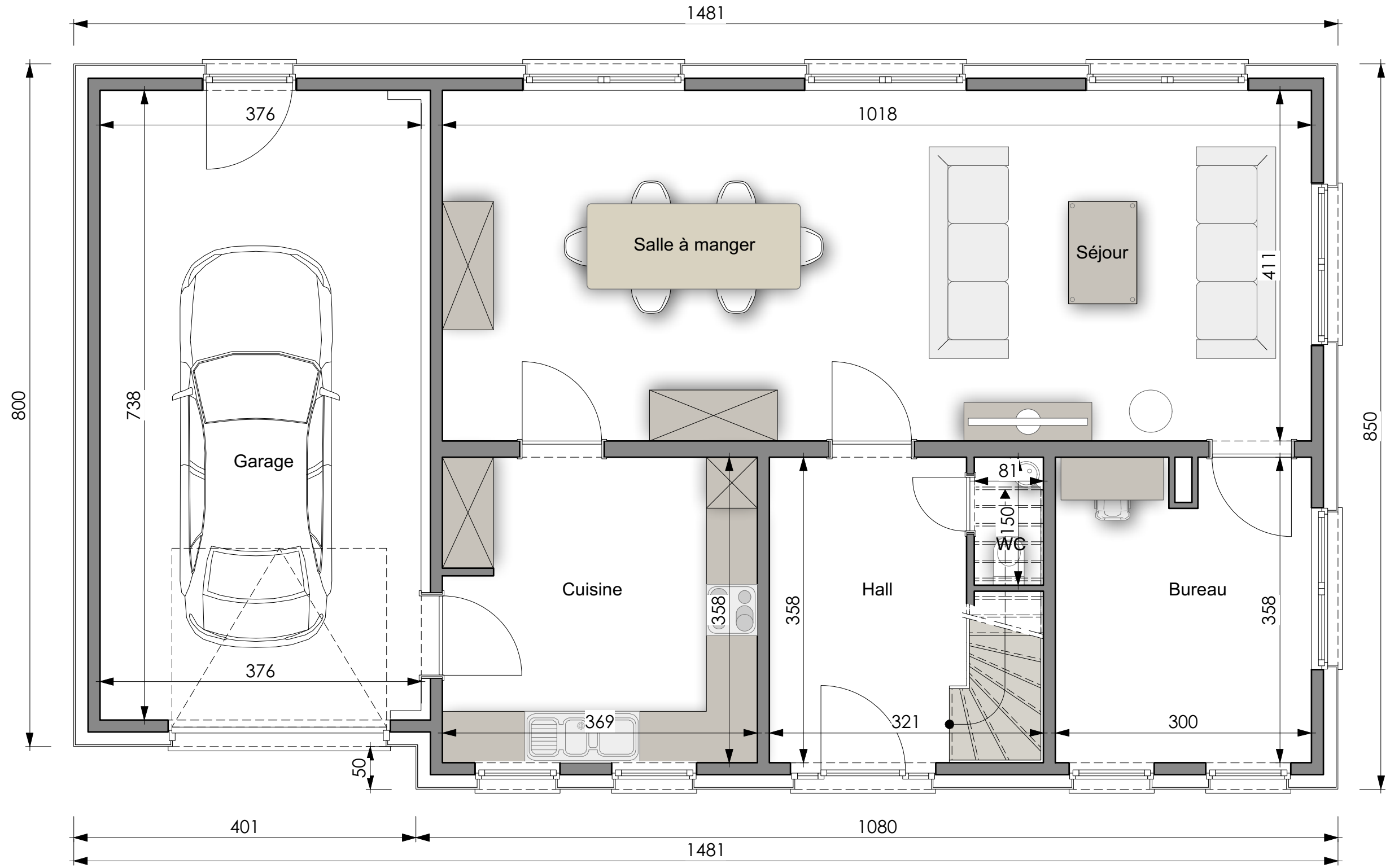
PLAN REZ-DE-CHAUSSEE
