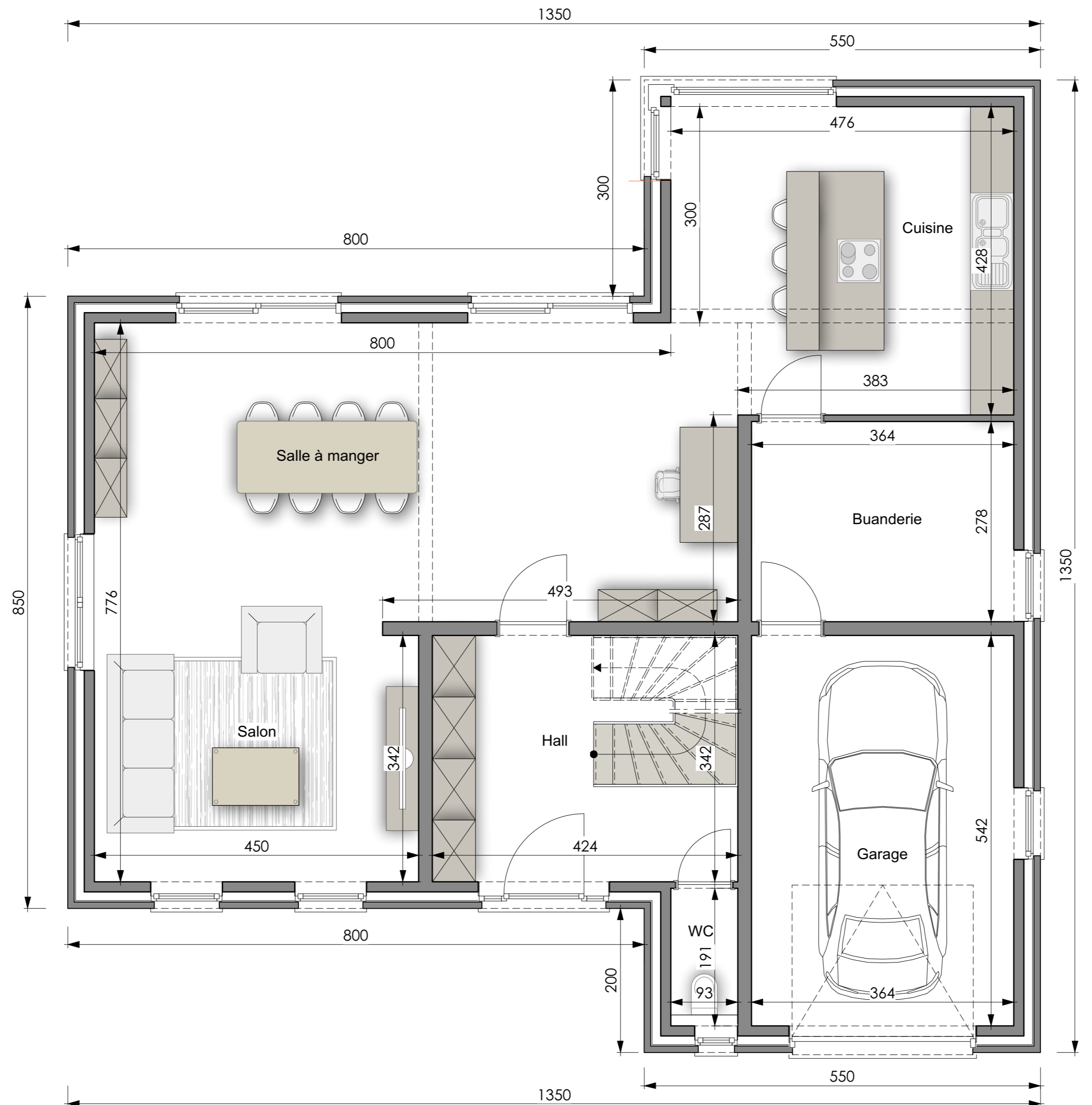
PLAN REZ-DE-CHAUSSEE
