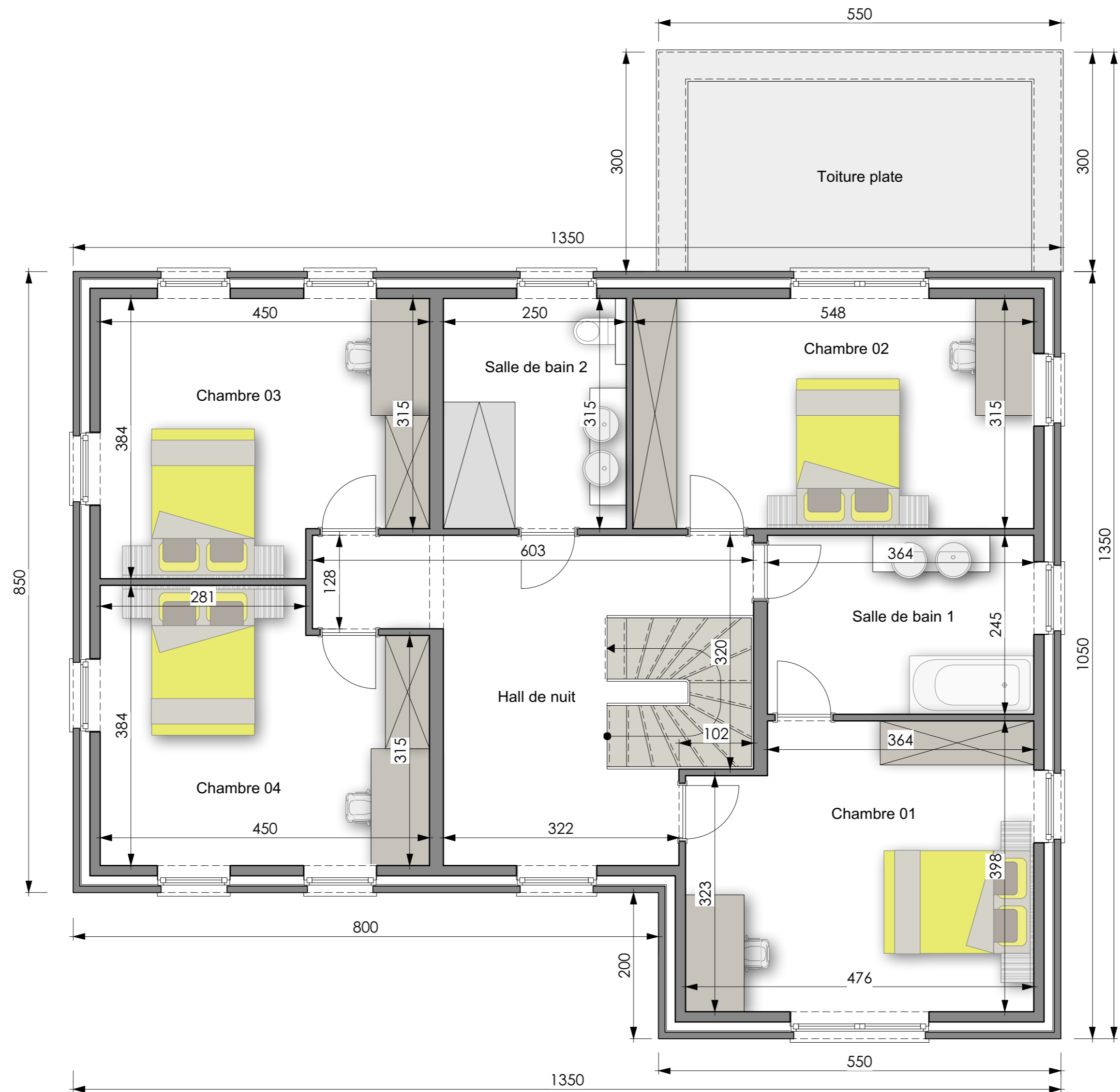
PLAN PREMIER ETAGE
